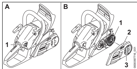
Kraftstoffhandpumpe (A)
